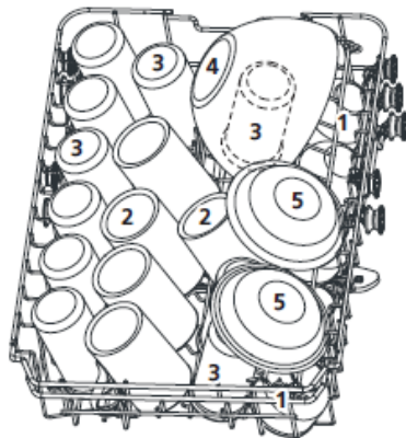
Cesta superior
